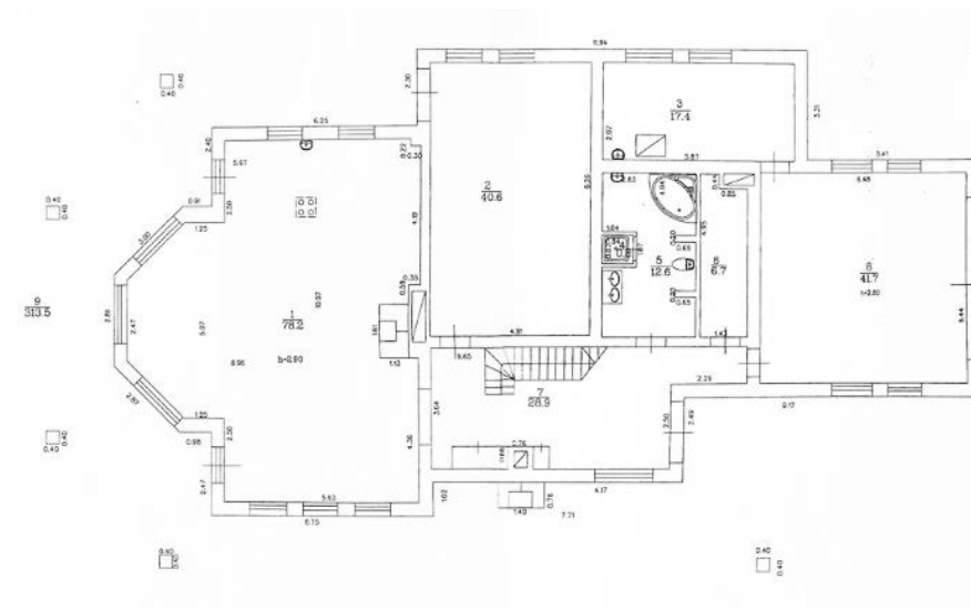
1. stāva plāns
